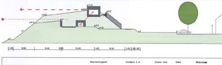
Principedetailering van verdedigingswerk in Hellevoetsluis.
